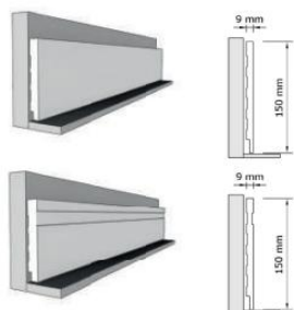
Liso | 150 x 2400mm
